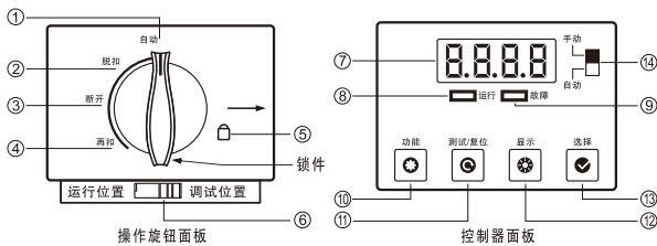
操作旋钮面板简介
